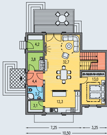
PRÍZEMIE [plocha 84.0 m 2 ]
