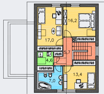
POSCHODIE [plocha 63.9 m 2 ]
