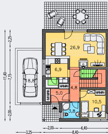
PRÍZEMIE [plocha 69.7 m 2 ]
