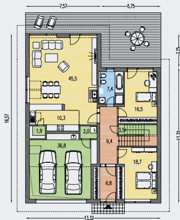
PRÍZEMIE [plocha 165.2 m 2 ]
