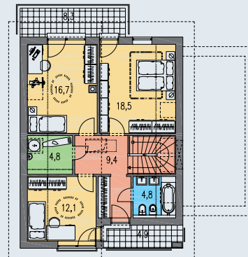
POSCHODIE [plocha 79.2 m 2 ]
