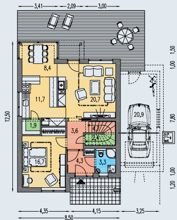
PRÍZEMIE [plocha 77.6 m 2 ]
