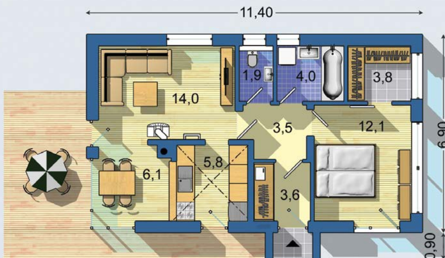
PRÍZEMIE [celková plocha 54.8 m 2 ]
