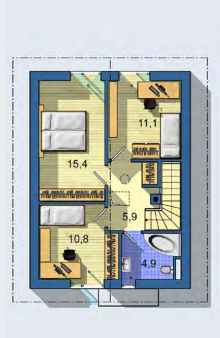
POSCHODIE [celková plocha 47.8 m 2 ]
