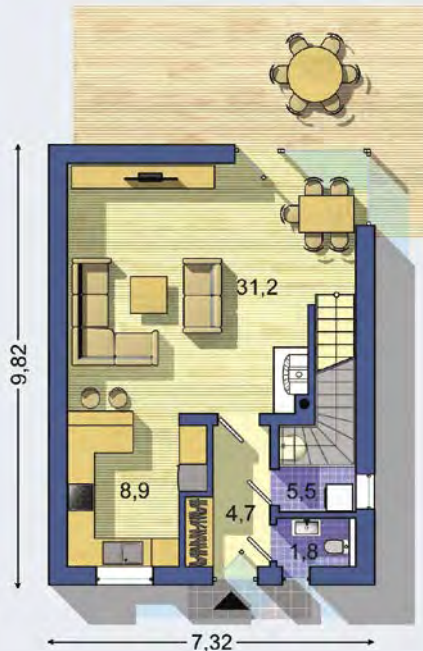
PRÍZEMIE [celková plocha 56.1 m 2 ]
