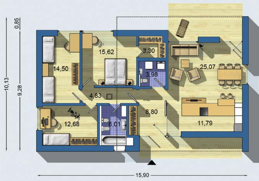
PRÍZEMIE [celková plocha 106.9 m 2 ]
