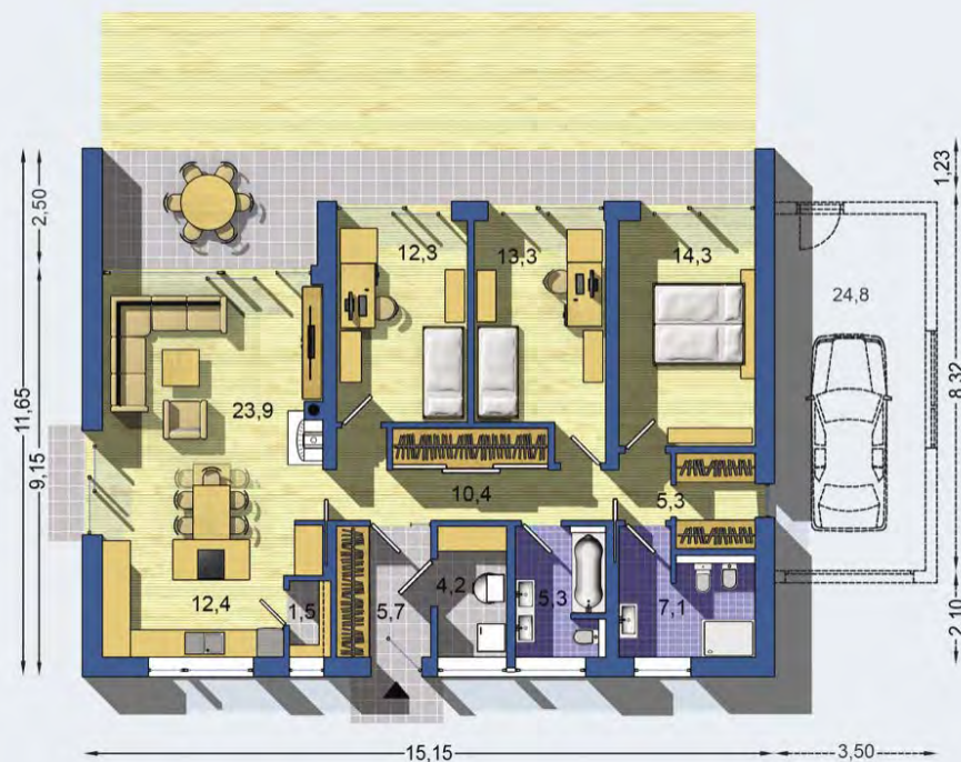
PRÍZEMIE [celková plocha 115.8 m 2 ]
